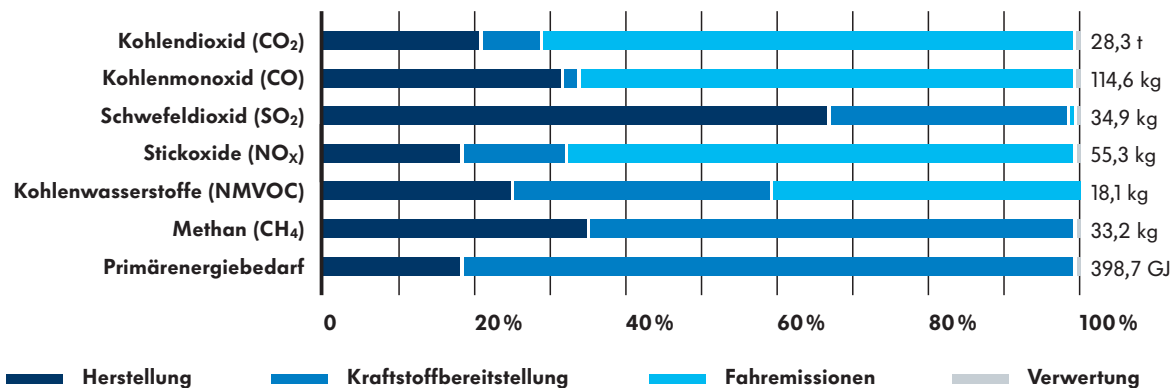
Abbildung 2: Sachbilanzdaten des Golf V 1,9 TDI [77kW] (Vorgänger)
