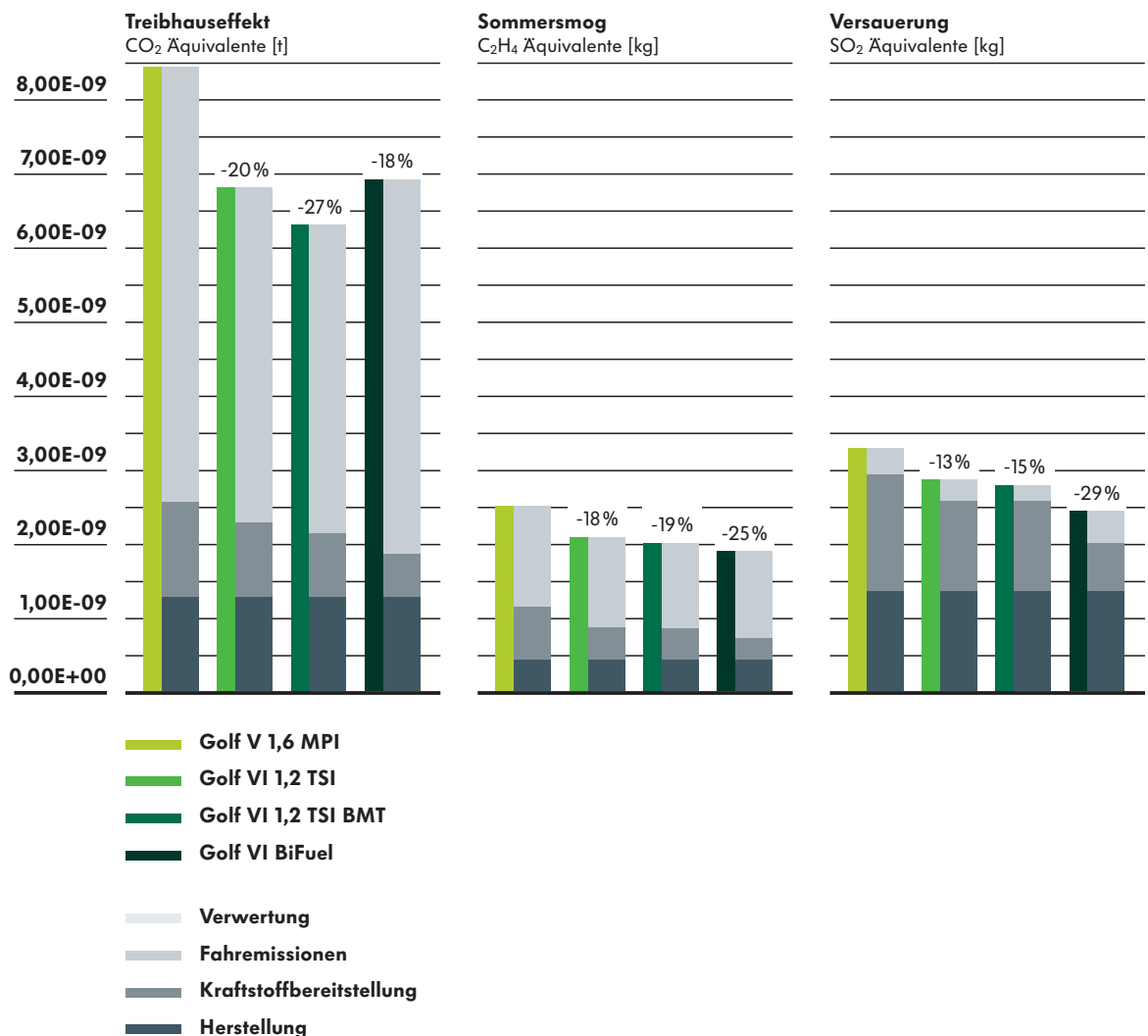
Abbildung 14: Umweltwirkungen des Benzin-Vorgängers und der Nachfolger Golf VI 1,2 TSI, 1,2 TSI BlueMotion Technology und Golf BiFuel (relativ)
