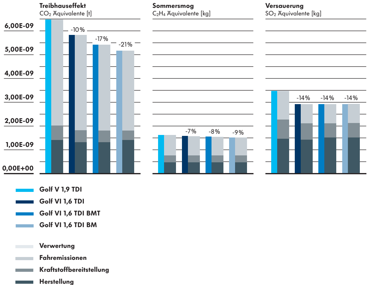
Abbildung 11: Umweltwirkungen Diesel-Vorgängers und der Nachfolger Golf VI 1,6 TDI, 1,6 TDI BlueMotion Technology und BlueMotion (relativ)
