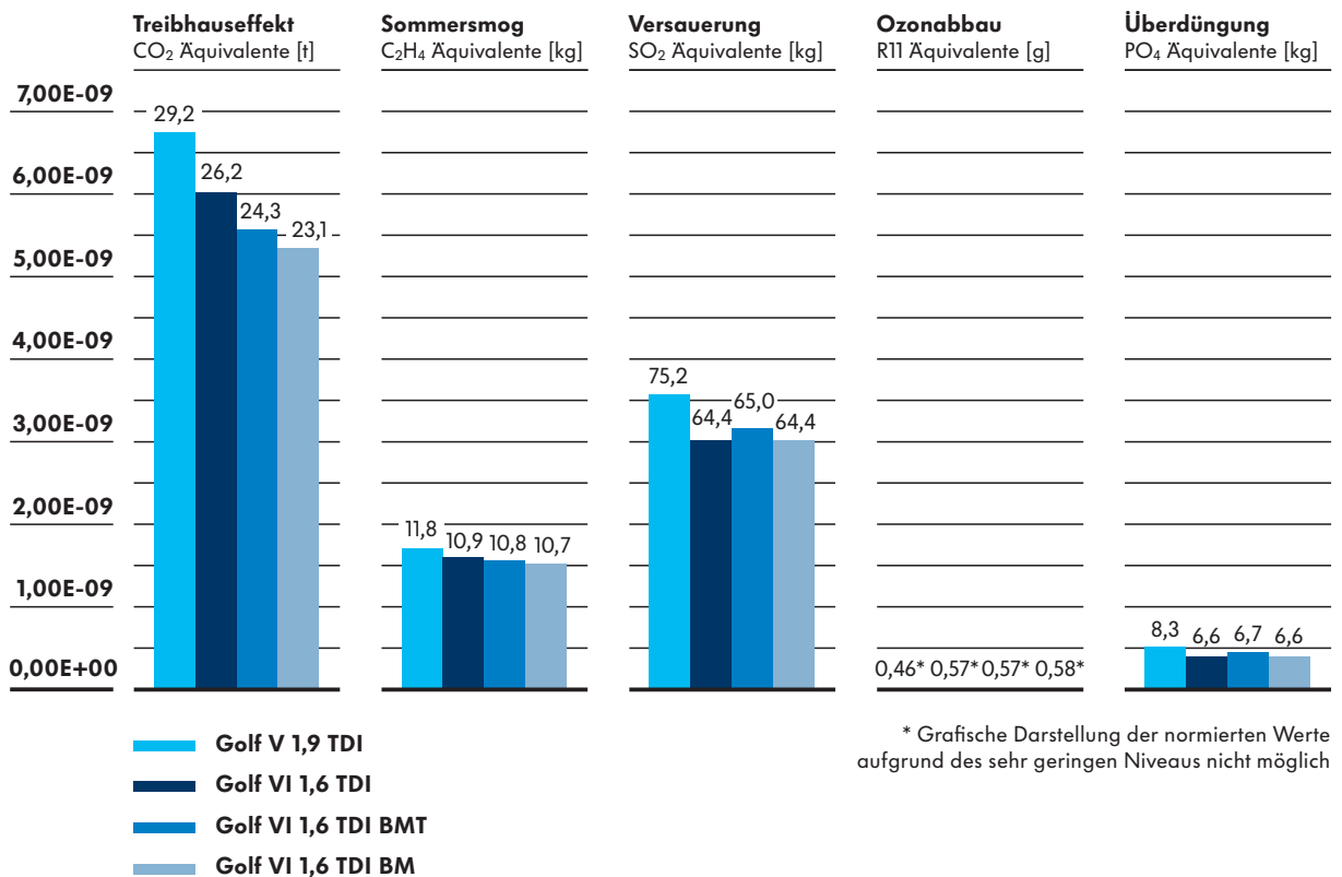
Abbildung 10: Umweltwirkungen von Golf V 1,9 TDI, Golf VI 1,6 TDI, 1,6 TDI BlueMotion Technology und BlueMotion (absolut)
