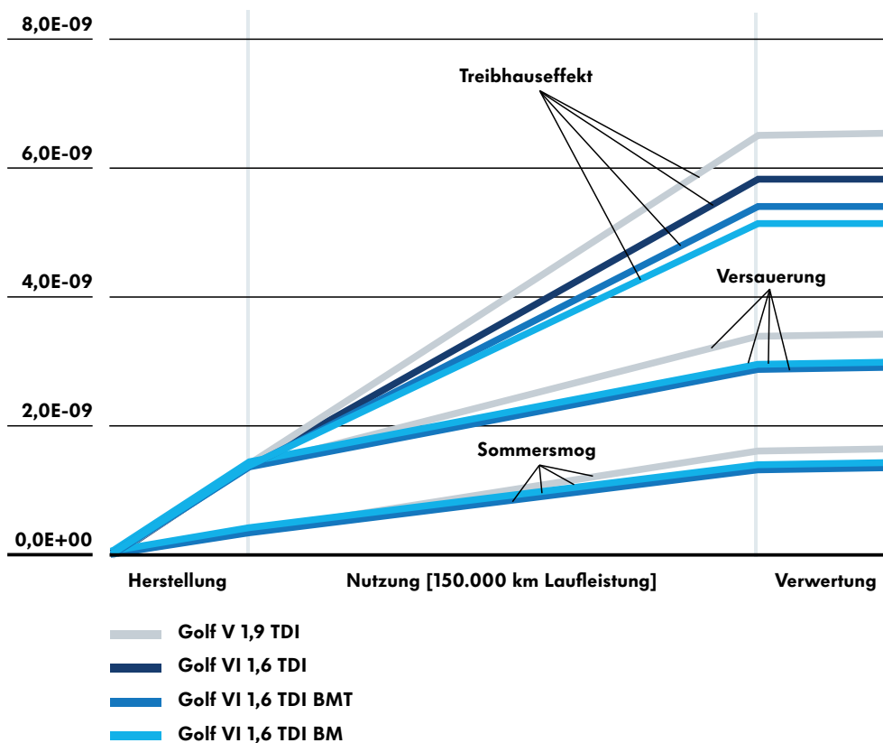
Abbildung 12: Vergleich der Umweltwirkungen über den Lebensweg – Dieselfahrzeuge
