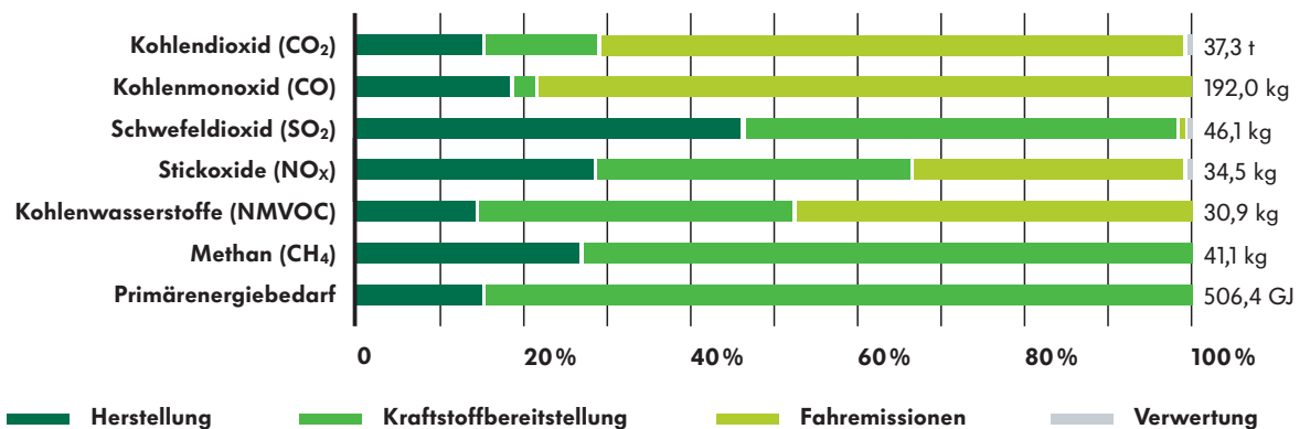
Abbildung 6: Sachbilanzdaten des Golf V 1,6 MPI [75kW] (Vorgänger)
