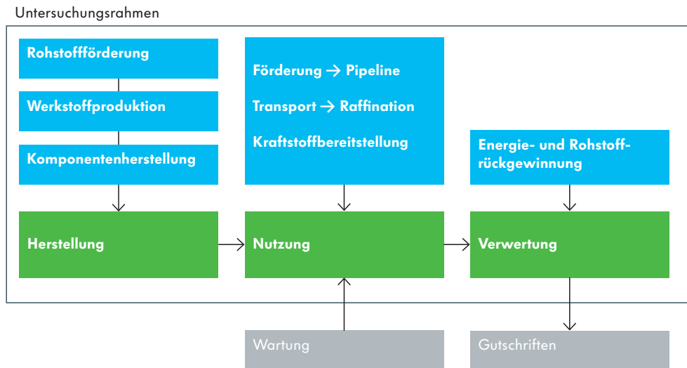
Abbildung 1: Untersuchungsrahmen der Umweltbilanz
