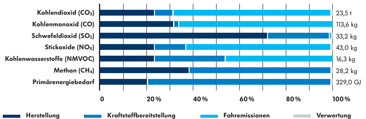
Abbildung 4: Sachbilanzdaten des Golf VI 1,6 TDI BlueMotion Technology [77kW]
