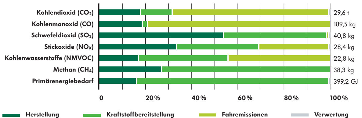
Abbildung 7: Sachbilanzdaten des Golf VI 1,2 TSI [77 kW]
