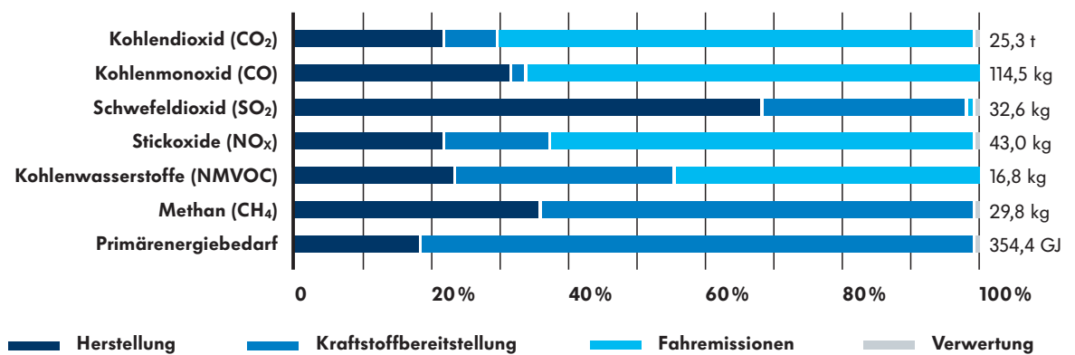
Abbildung 3: Sachbilanzdaten des Golf VI 1,6 TDI [77 kW]
