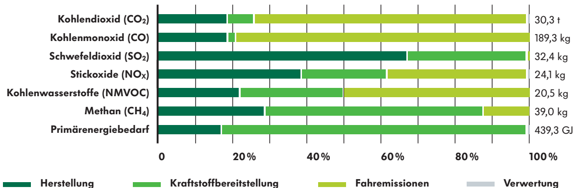
Abbildung 9: Sachbilanzdaten des Golf VI BiFuel [75 kW/ 72 kW]
