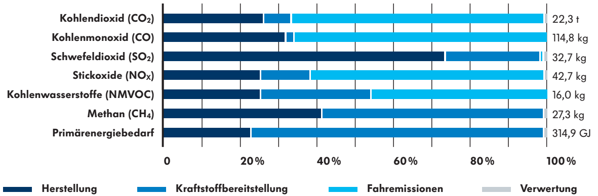
Abbildung 5: Sachbilanzdaten des Golf VI 1,6 TDI BlueMotion [77kW]
