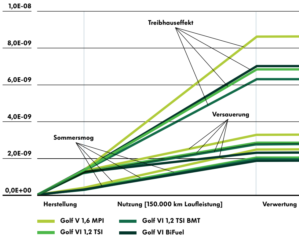
Abbildung 15: Vergleich der Umweltwirkungen über den Lebensweg – Benzinerfahrzeuge
