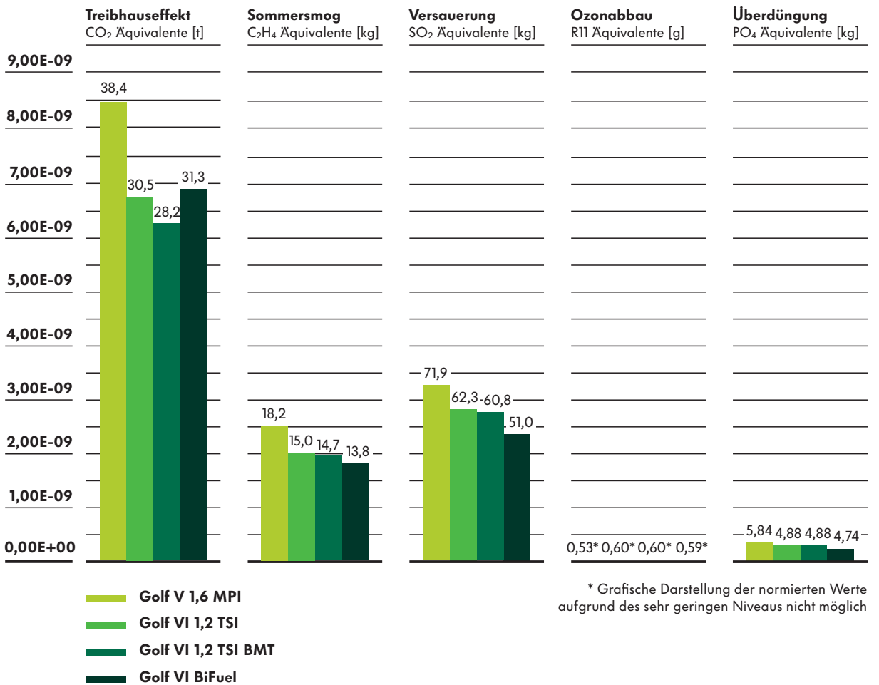
Abbildung 13: Umweltwirkungen von Golf V 1,6 MPI (Vorgänger), Golf VI 1,2 TSI, 1,2 TSI BlueMotion Technology und BiFuel (absolut)
