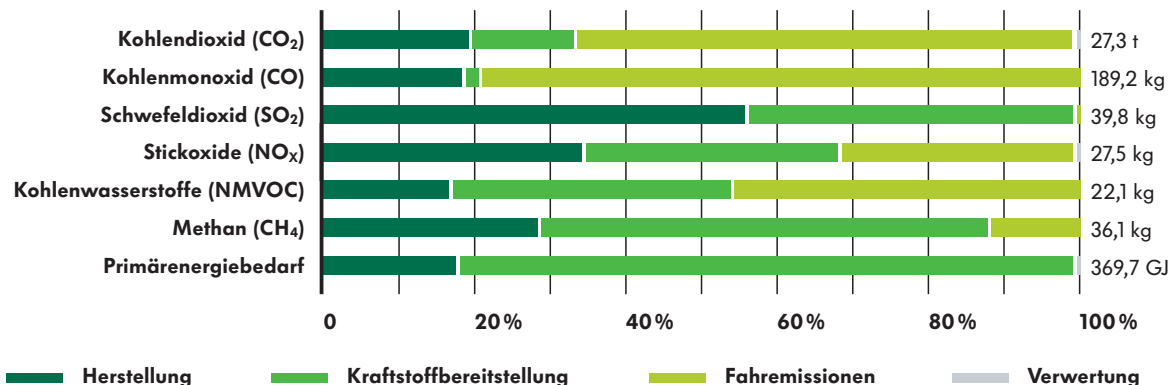
Abbildung 8: Sachbilanzdaten des Golf VI 1,2 TSI BlueMotion Technology [77 kW]
